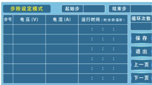
步阶设置页面可设置所需电压、电流运行时间、初始步、结束步和循环次数
